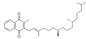
维生素 K 1 (M.W. 450.71)
